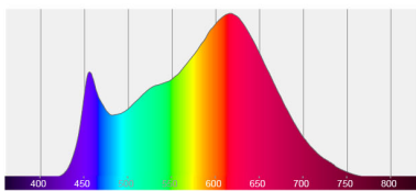
Spectra
