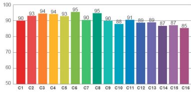
TM30: 91.0
